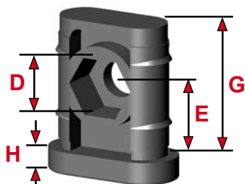
3D1BO30X15X1.5M8F/0
