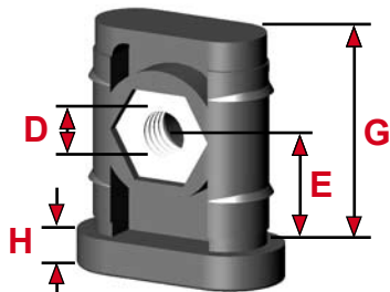
3D1BO30X15X1.5M8F/1
