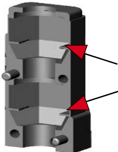
DIN 985 M8/M10 oder/or/ou DIN 934 M8/M10
